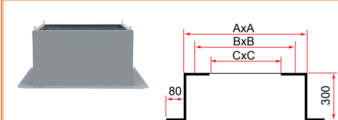
Costière toit plat en acier galvanisé
