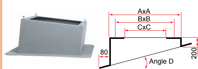
Costière toit incliné en acier galvanisé
