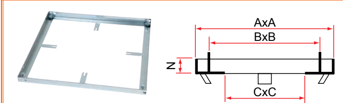
Cadre à sceller en acier galvanisé
