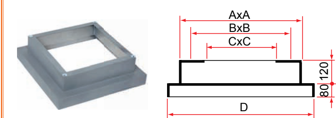
Costière souche maçonnée en acier galvanisé
